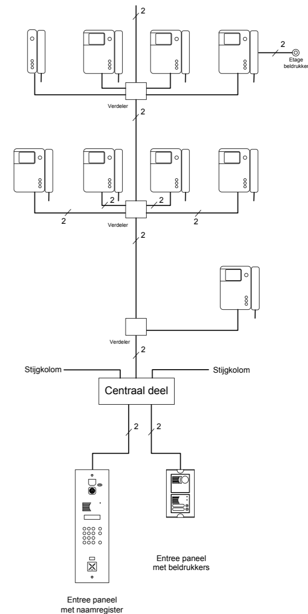
2 VOICE (Verdeling met videoverdelers)
